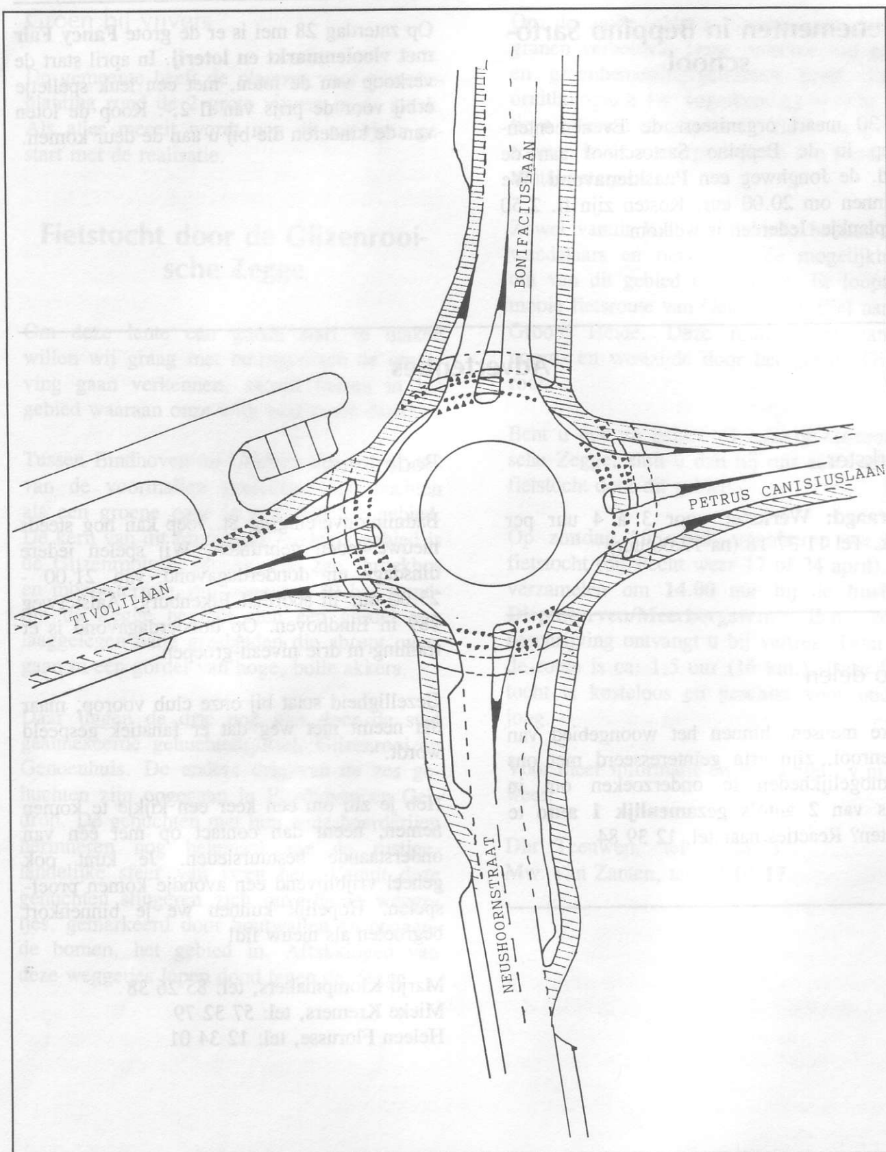
Situatieschets mini-rotonde Tivolilaan/Neushoornstraat
